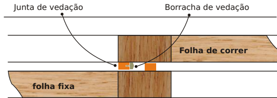
Vista Superior - janela de correr
