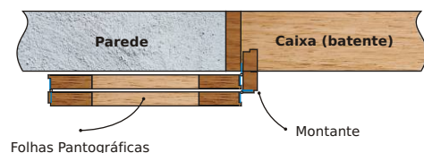
detalhe da pantográfica de remontar
