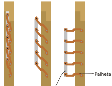
Barra de alumínio Palheta Montante detalhe da veneziana móvel
