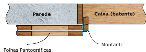
detalhe da pantográfica de remontar
